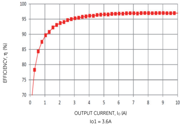
Fig 9a: Efficiency
