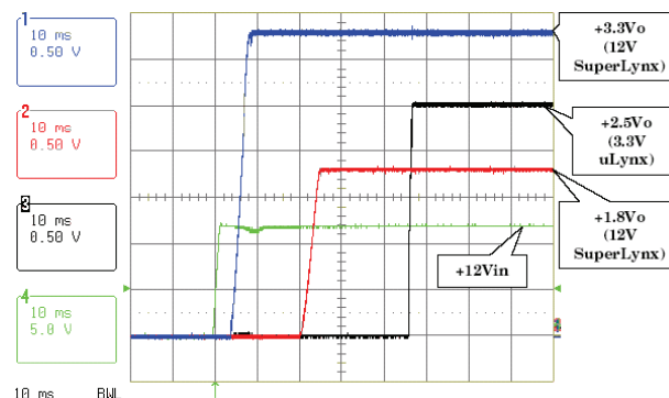
Fig. 5 Test Data
