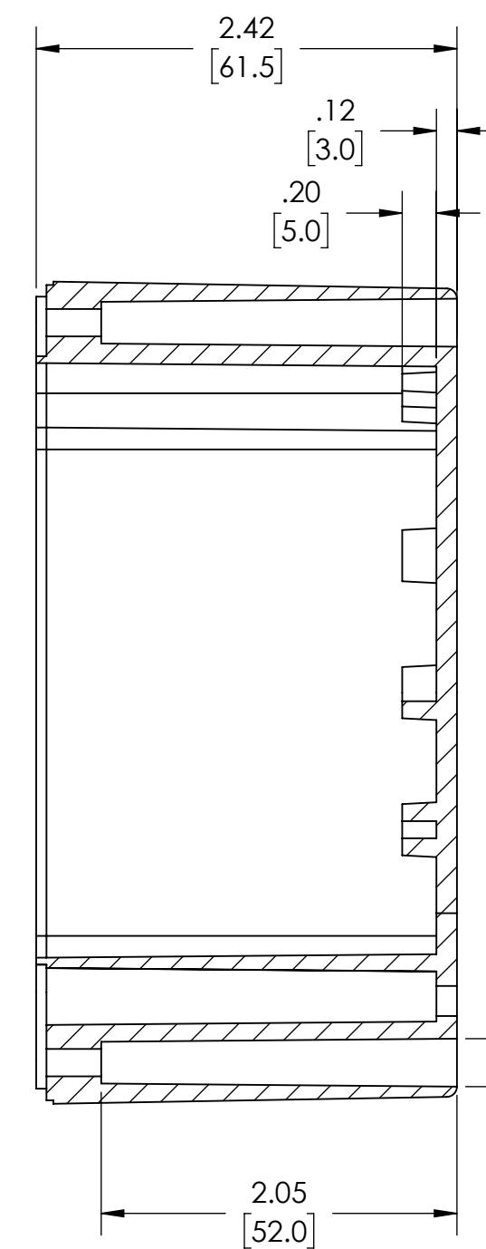
SECTION A-A
