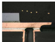
Thermal Via
