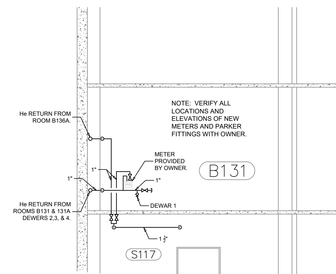
ELEVATION DD SCALE: 1/8" = 1'-0"
