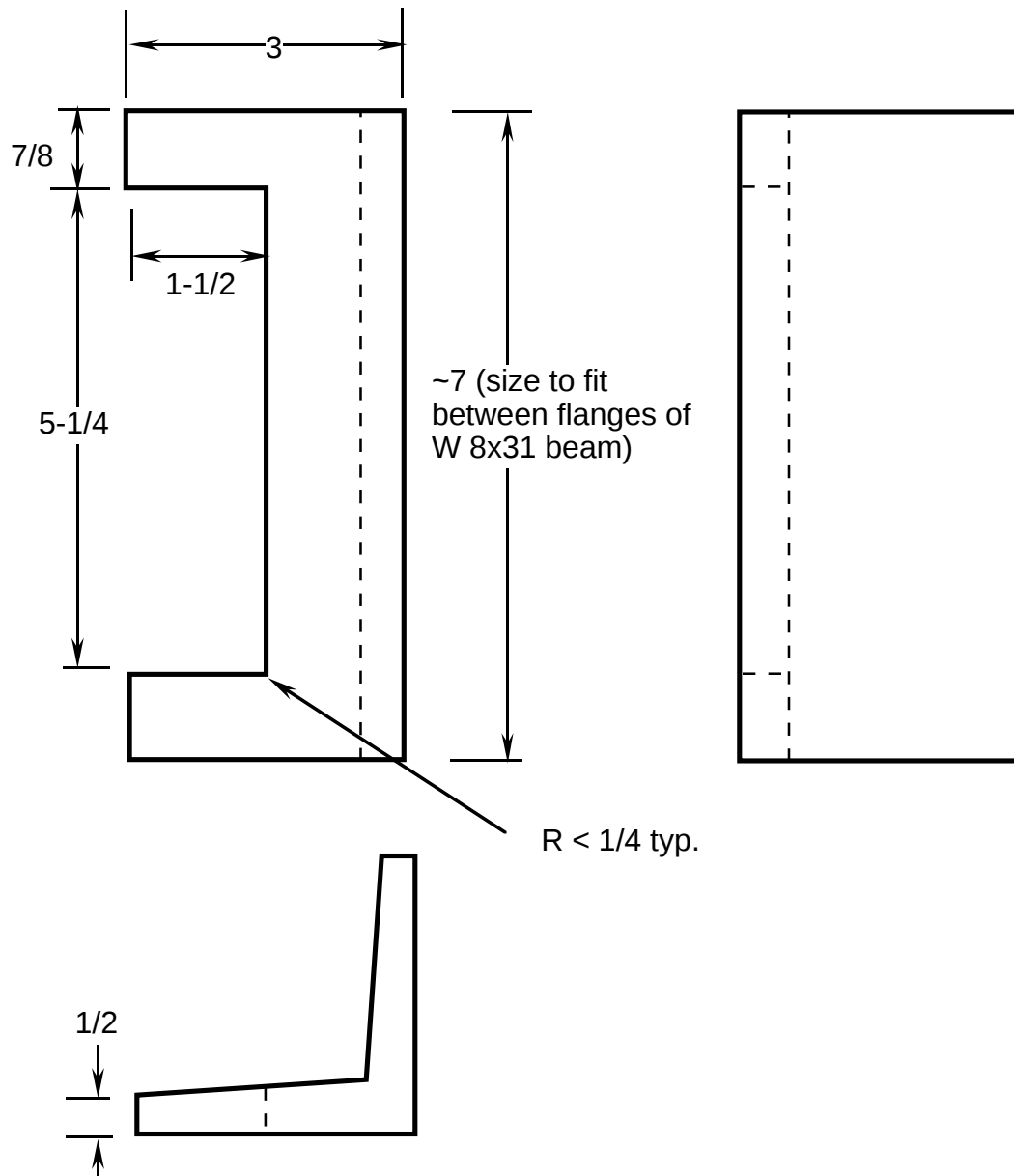
END GUSSET
